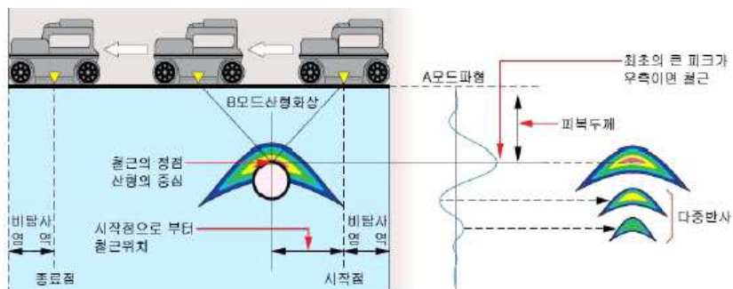
<그림 3.52> RC-Radar 원리
